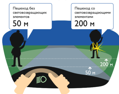
Ближний свет фар
